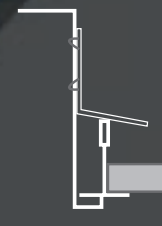
Perfilería vista, luminaria semi-empotrada
