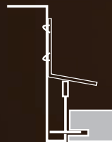
Perfilería "T" oculta, techo no desmontable
