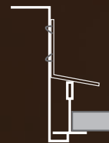
Perfilería vista, luminaria semi-empotrada
